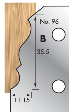
Cutter: 003H00096 Limiter: 004H00096
