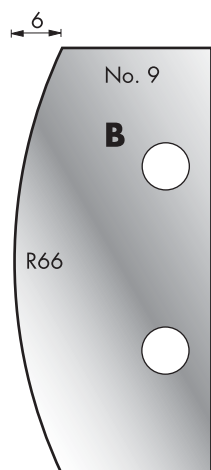
Cutter: 003H00009 Limiter: 004H00009
