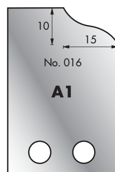
Cutter: 005H00016 Limiter: 006H00016
