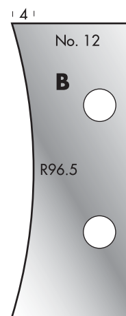
Cutter: 003H00012 Limiter: 004H00012
