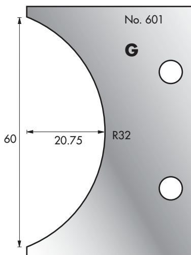
Cutter: 003H00601 Limiter: 004H00601
