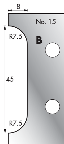
Cutter: 003H00015 Limiter: 004H00015
