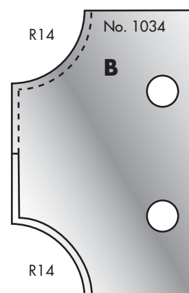
Cutter: 003H01034 Limiter: 004H01034
