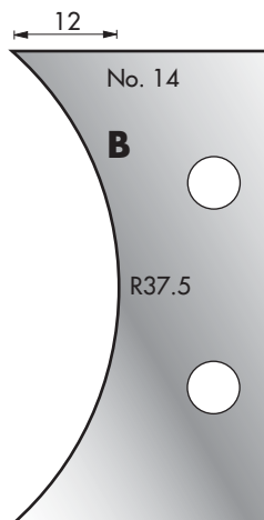
Cutter: 003H00014 Limiter: 004H00014
