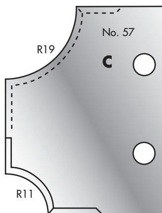
Cutter: 003H00057 Limiter: 004H00057
