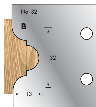
Cutter: 003H00082 Limiter: 004H00082
