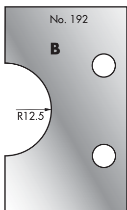
Cutter: 003H00192 Limiter: 004H00192
