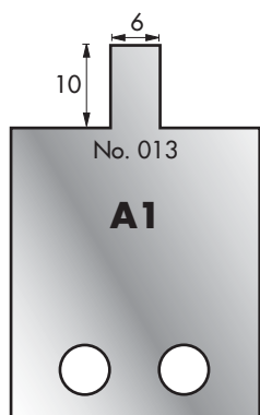
Cutter: 005H00013 Limiter: 006H00013
