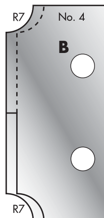
Cutter: 003H00004 Limiter: 004H00004
