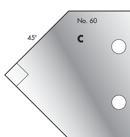
Cutter: 003H00060 Limiter: 004H00060
