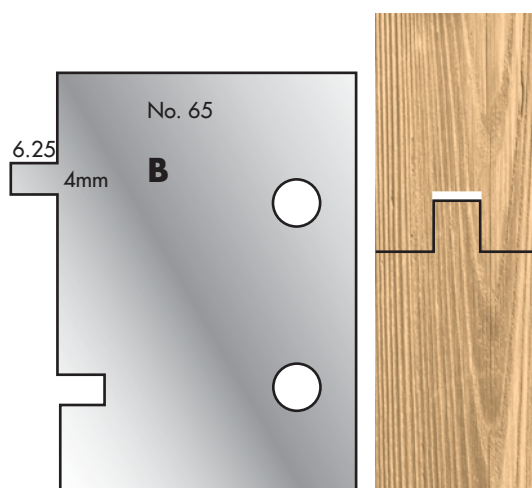
Cutter: 003H00065 Limiter: 004H00065
