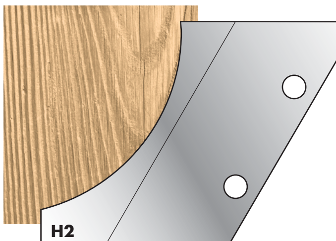
Cutter: 003H000H2 Limiter: 004H000H2
