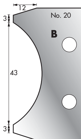
Cutter: 003H00020 Limiter: 004H00020
