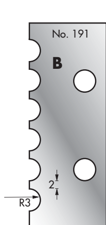
Cutter: 003H00191 Limiter: 004H00191
