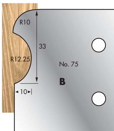
Cutter: 003H00075 Limiter: 004H00075
