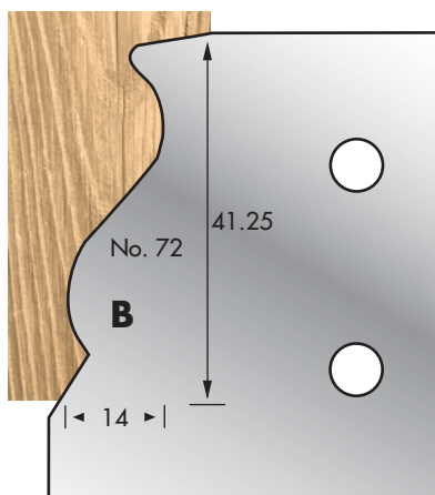
Cutter: 003H00072 Limiter: 004H00072
