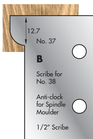
Cutter: 003H00037 Limiter: 004H00037
