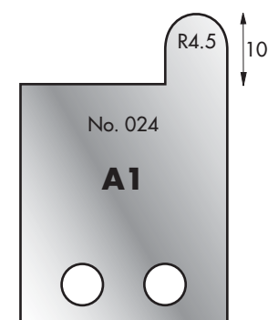
Cutter: 005H00024 Limiter: 006H00024
