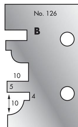
Cutter: 003H00126 Limiter: 004H00126
