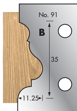
Cutter: 003H00091 Limiter: 004H00091
