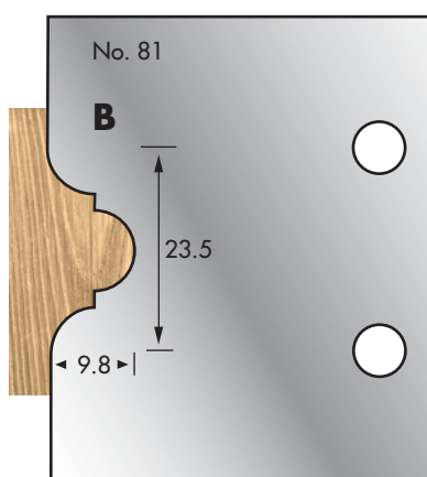
Cutter: 003H00081 Limiter: 004H00081
