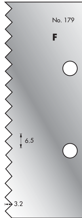
Cutter: 003H00179 Limiter: 004H00179
