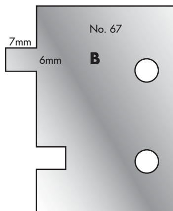
Cutter: 003H00067 Limiter: 004H00067
