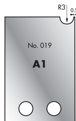
Cutter: 005H00019 Limiter: 006H00019
