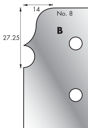
Cutter: 003H00008 Limiter: 004H00008
