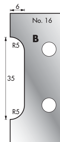
Cutter: 003H00016 Limiter: 004H00016
