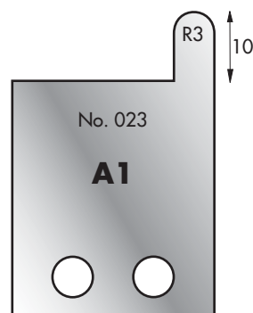
Cutter: 005H00023 Limiter: 006H00023
