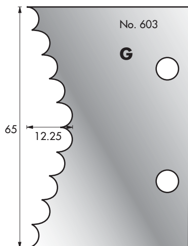
Cutter: 003H00603 Limiter: 004H00603
