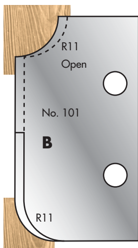
Cutter: 003H00101 Limiter: 004H00101
