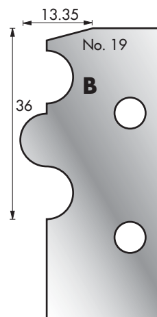
Cutter: 003H00019 Limiter: 004H00019
