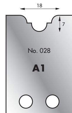
Cutter: 005H00028 Limiter: 006H00028
