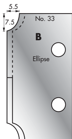
Cutter: 003H00033 Limiter: 004H00033
