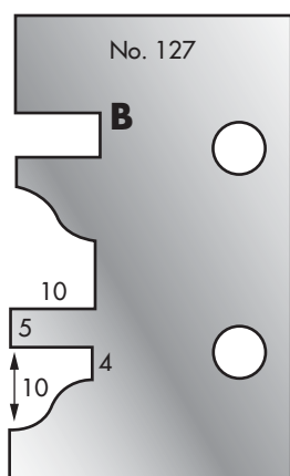
Cutter: 003H00127 Limiter: 004H00127
