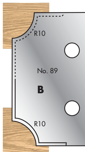
Cutter: 003H00089 Limiter: 004H00089
