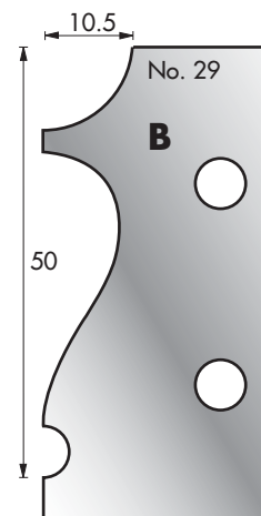
Cutter: 003H00029 Limiter: 004H00029
