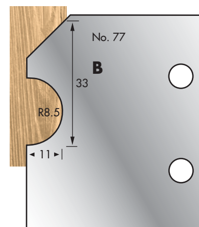
Cutter: 003H00077 Limiter: 004H00077
