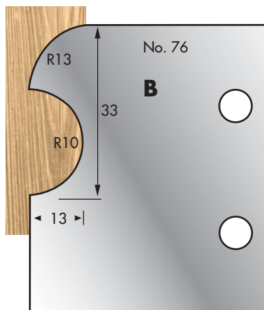
Cutter: 003H00076 Limiter: 004H00076
