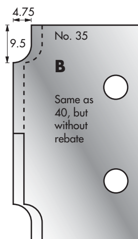
Cutter: 003H00035 Limiter: 004H00035
