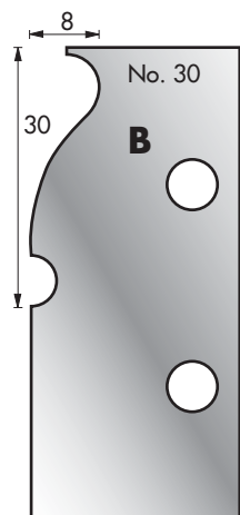
Cutter: 003H00030 Limiter: 004H00030
