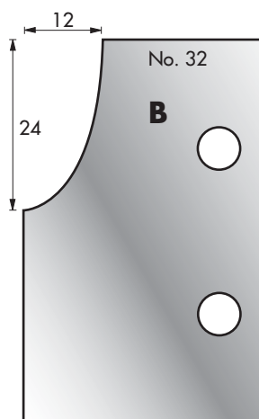
Cutter: 003H00032 Limiter: 004H00032
