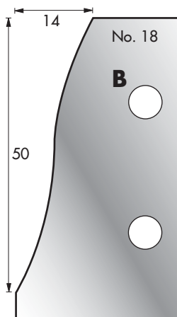
Cutter: 003H00018 Limiter: 004H00018
