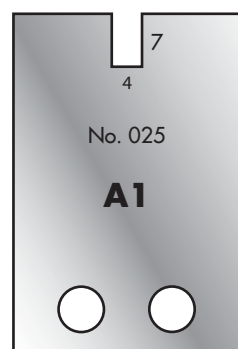
Cutter: 005H00025 Limiter: 006H00025
