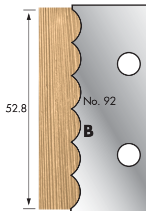
Cutter: 003H00092 Limiter: 004H00092
