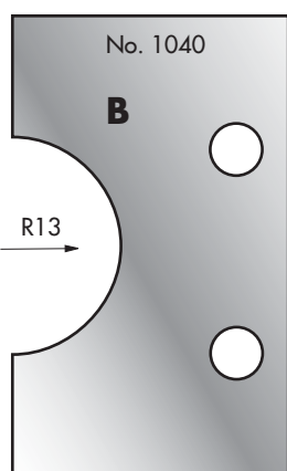
Cutter: 003H01040 Limiter: 004H01040
