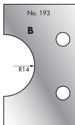
Cutter: 003H00193 Limiter: 004H00193
