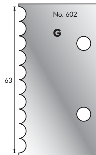
Cutter: 003H00602 Limiter: 004H00602
