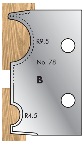
Cutter: 003H00078 Limiter: 004H00078
