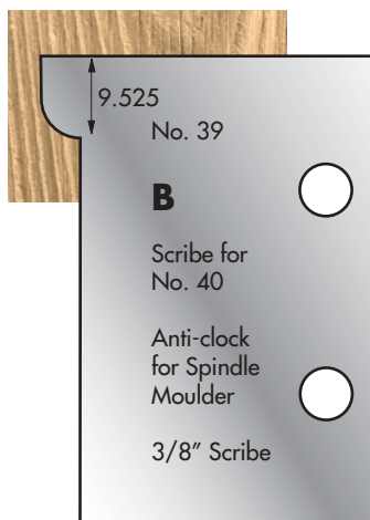
Cutter: 003H00039 Limiter: 004H00039
