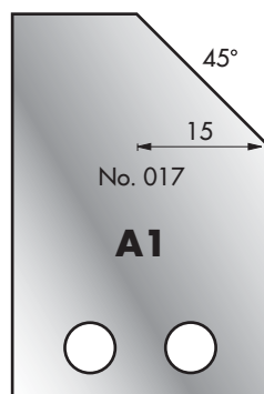
Cutter: 005H00017 Limiter: 006H00017
