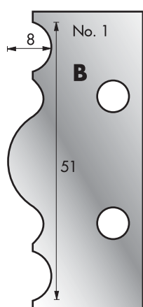
Cutter: 003H00001 Limiter: 004H00001
