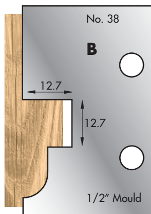
Cutter: 003H00038 Limiter: 004H00038
