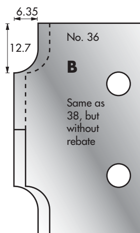
Cutter: 003H00036 Limiter: 004H00036
