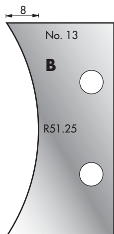
Cutter: 003H00013 Limiter: 004H00013
