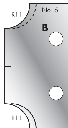
Cutter: 003H00005 Limiter: 004H00005
