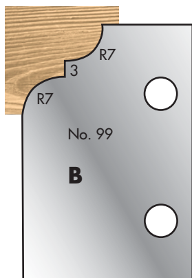
Cutter: 003H00099 Limiter: 004H00099
