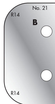
Cutter: 003H00021 Limiter: 004H00021
