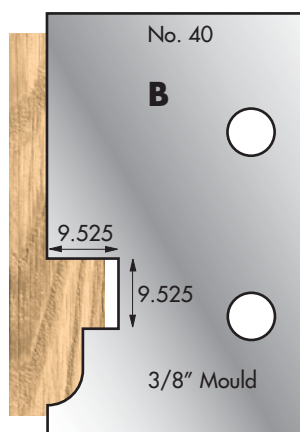
Cutter: 003H00040 Limiter: 004H00040
