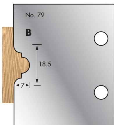
Cutter: 003H00079 Limiter: 004H00079
