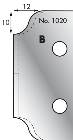
Cutter: 003H01020 Limiter: 004H01020
