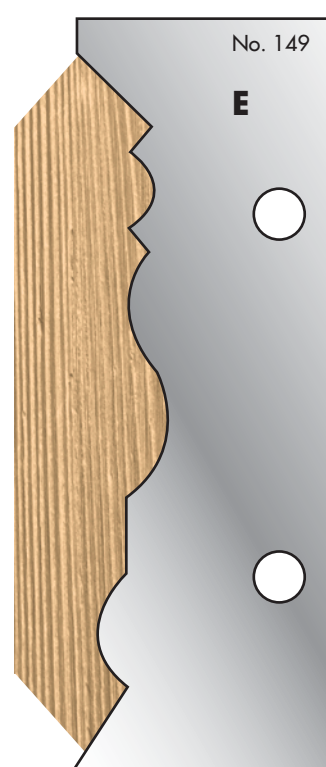
Cutter: 003H00149 Limiter: 004H00149
