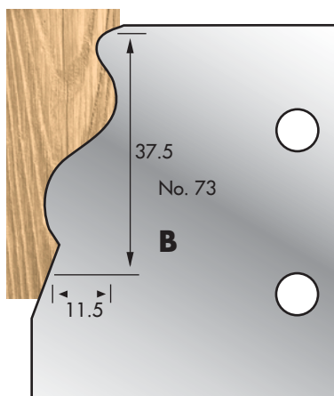
Cutter: 003H00073 Limiter: 004H00073
