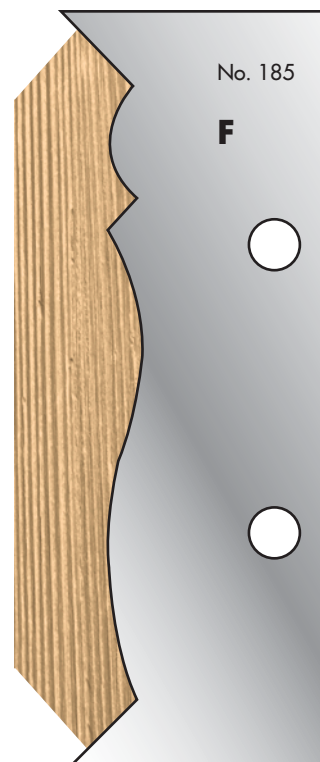
Cutter: 003H00185 Limiter: 004H00185
