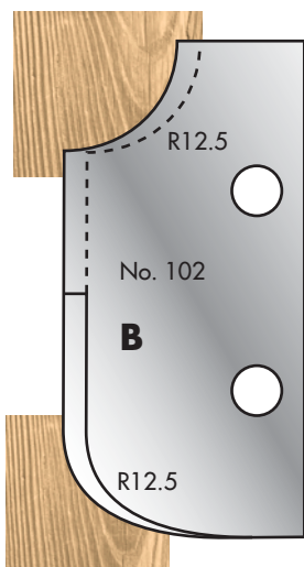
Cutter: 003H00102 Limiter: 004H00102
