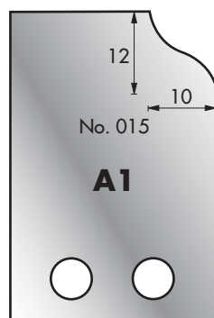
Cutter: 005H00015 Limiter: 006H00015
