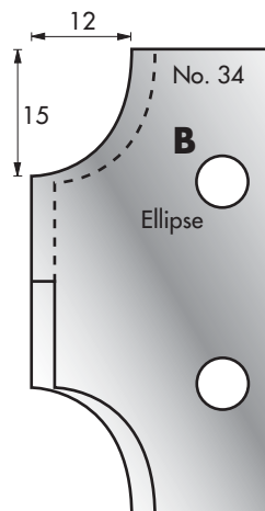
Cutter: 003H00034 Limiter: 004H00034
