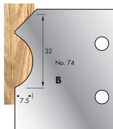
Cutter: 003H00074 Limiter: 004H00074
