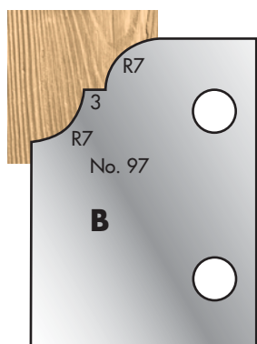
Cutter: 003H00097 Limiter: 004H00097
