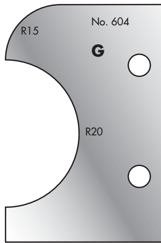
Cutter: 003H00604 Limiter: 004H00604
