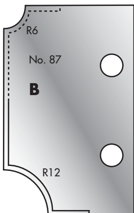
Cutter: 003H00087 Limiter: 004H00087
