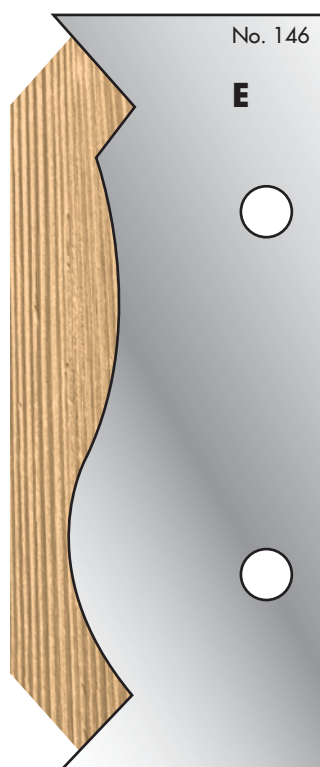
Cutter: 003H00146 Limiter: 004H00146
