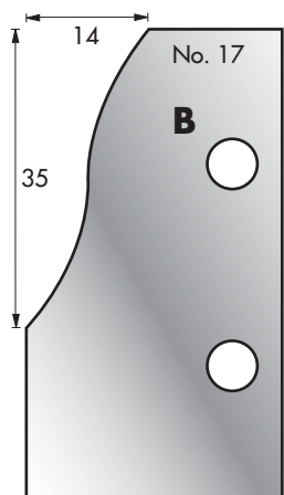
Cutter: 003H00017 Limiter: 004H00017
