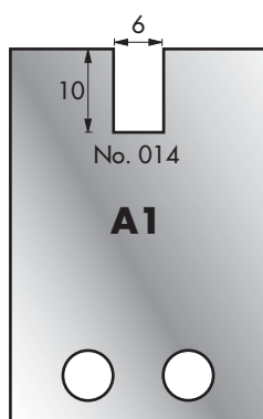
Cutter: 005H00014 Limiter: 006H00014
