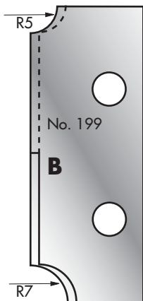
Cutter: 003H00199 Limiter: 004H00199
