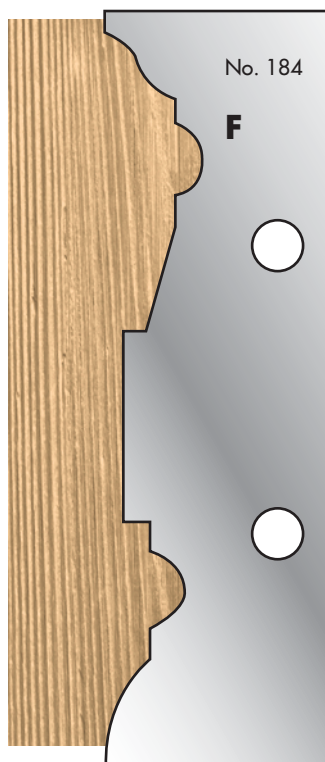
Cutter: 003H00184 Limiter: 004H00184
