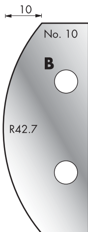
Cutter: 003H00010 Limiter: 004H00010
