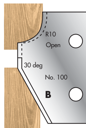
Cutter: 003H00100 Limiter: 004H00100
